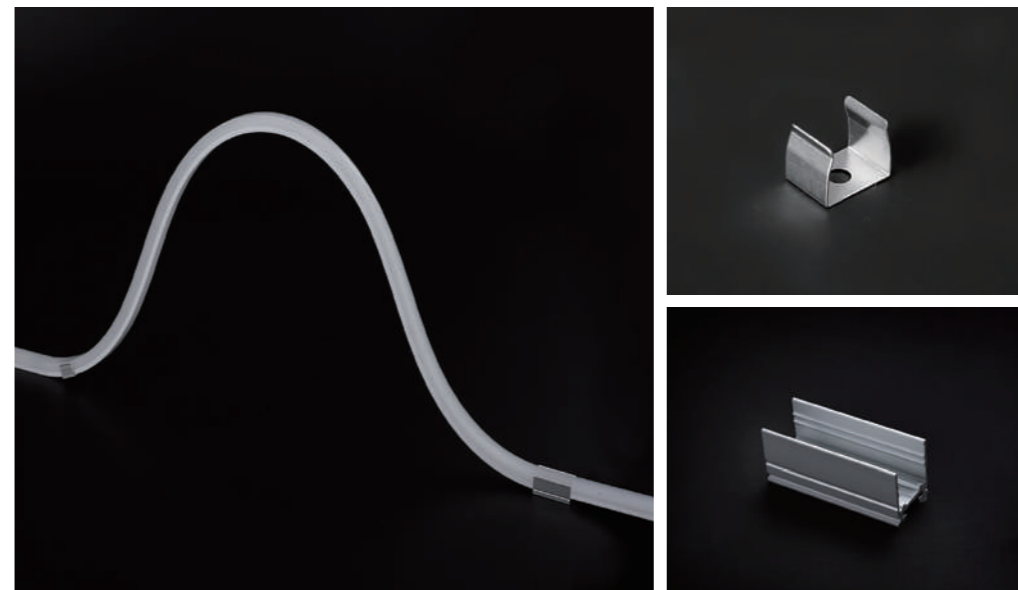
Stainless Clips Item No : JK0015 Dimension(LxWxH) : 15 X 17 X 8.8mm Material : SUS304,SUS316
